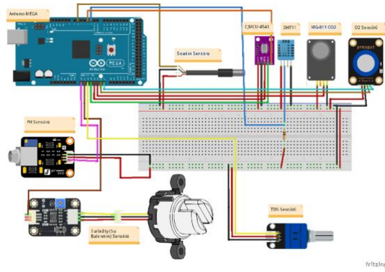
Şekil 3: Devre tasarımı
