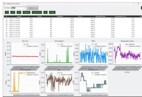
Şekil 4: Biyoreaktörler için geliştirilen test sistemi arayüzü
